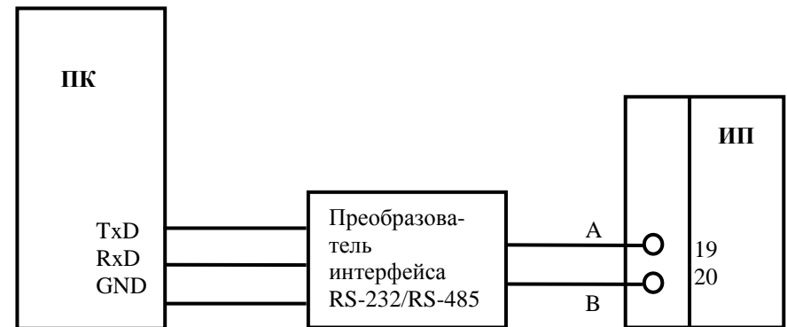
Рисунок 1- Подключение ИП к персональному компьютеру
